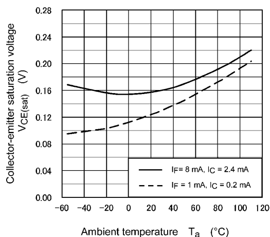
Fig. 11.12 V_{CE(sat)} - T_a
