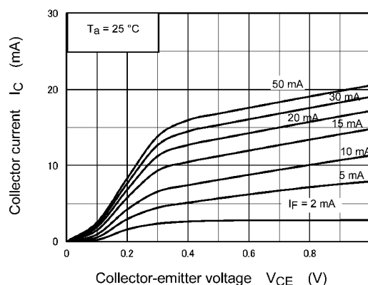
Fig. 11.8 I_C - V_{CE}
