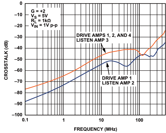
图38. ADA4851-4 RTI串扰与频率的关系
