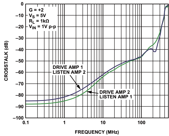
图39. ADA4851-2 RTI串扰与频率的关系
