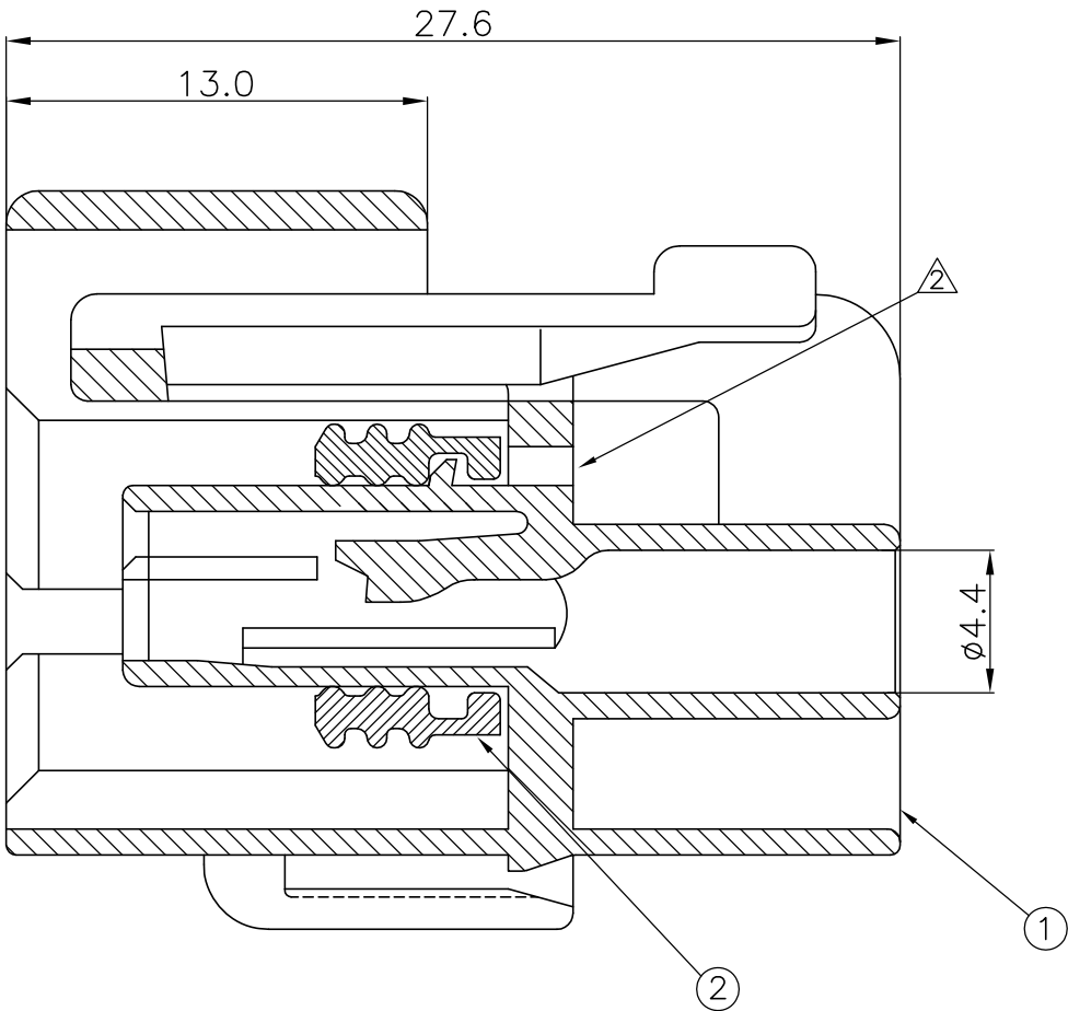
SECT A-A
