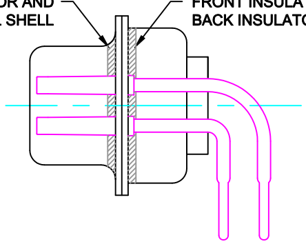
DETAIL A-A
