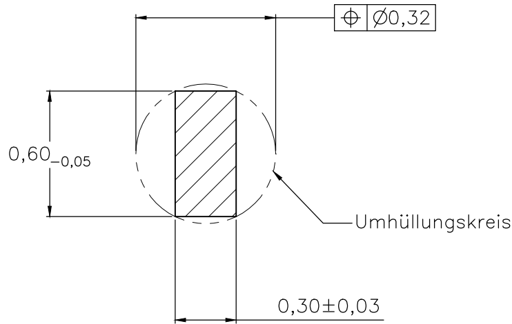
Schnitt AB des Lötanschlusses Cross-section AB of solderpin (20:1)
