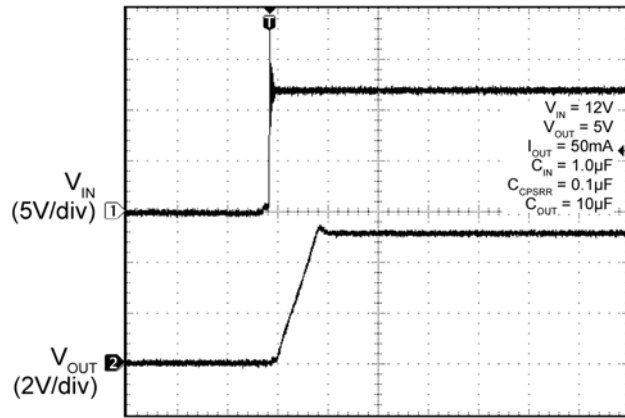
Fast Turn-On
