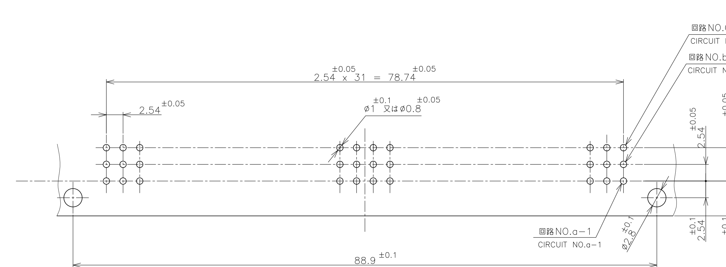
P.C. BOARD LAYOUT DIMENSIONS プリント基板 取付寸法 (コネクタ搭載面)
