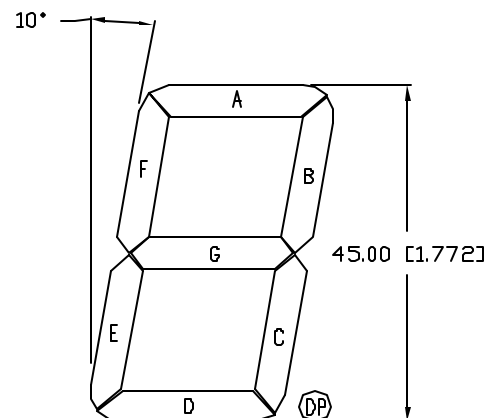
DIGIT DETAIL
