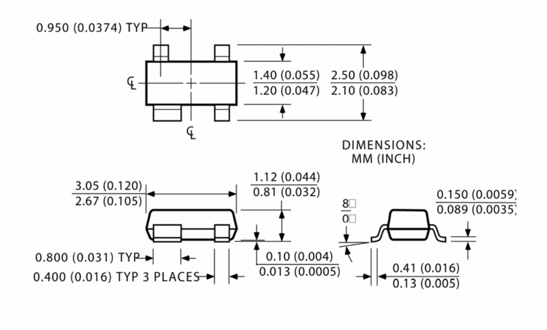
SOT-143 (M4)
