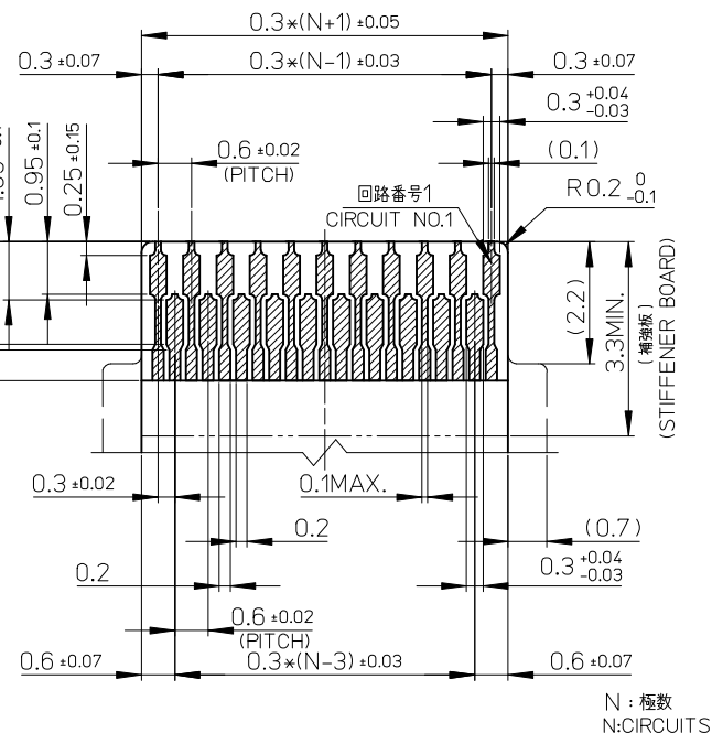
適合する金めっきFPC推奨寸法 APPLICABLE FPC OF GOLD PATING RECOMMENDED DIMENSION (仕上がり厚さ: 0.2 ± 0.03) (THICKNESS: 0.2 ± 0.03)
