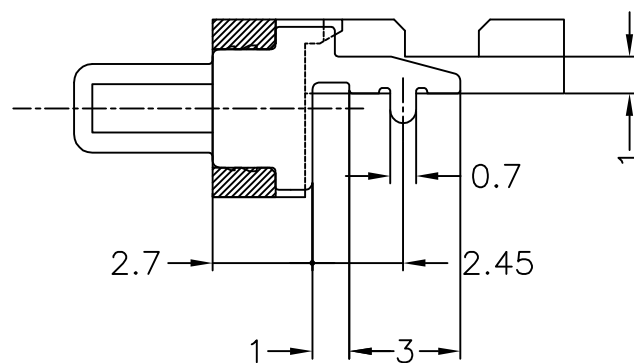
SECT."A"—"A" (SCALE:5-1)
