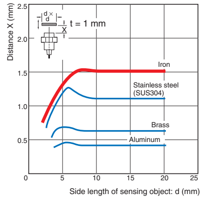
E2E-X10E/-X10Y/-X10F
