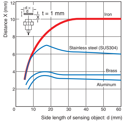
E2E-X10ME/-X10MY/-X10MF
