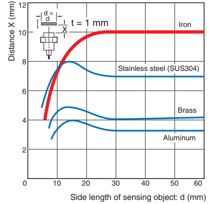
E2E-X10ME/-X10MY/-X10MF
