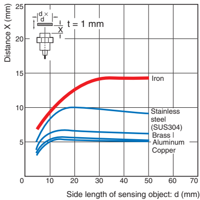
E2E-X2E/-X2Y/-X2F
