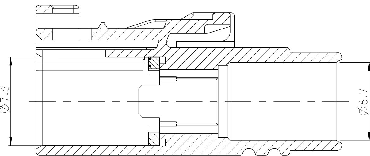
A-A
