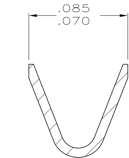
SECTION A-A SCALE 20:1
