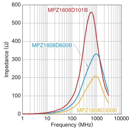
MPZ1608D 系列
