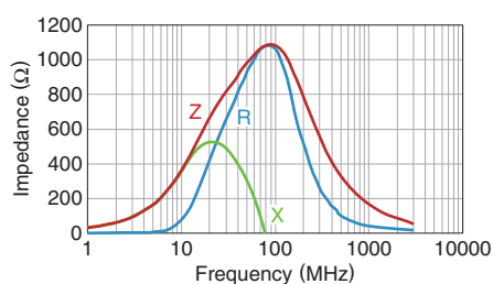
MMZ2012S102AT000
