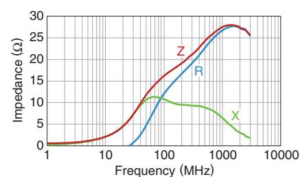
MMZ2012Y150BT000
