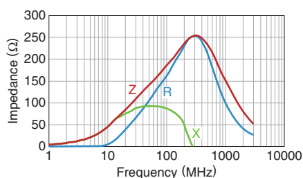
MMZ2012S181AT000
