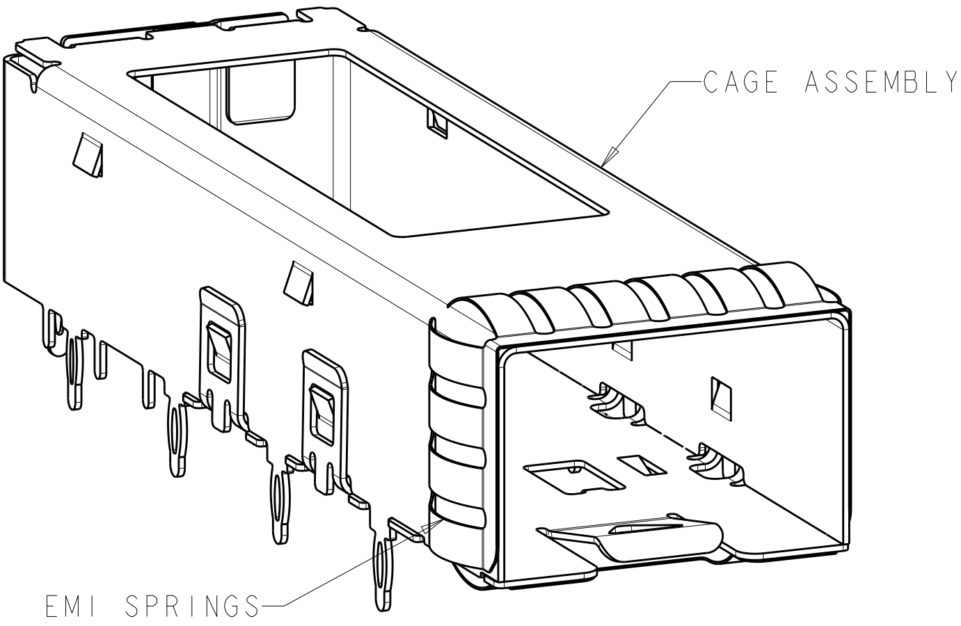
2007215-2 SCALE 5:1
