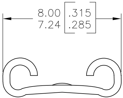
VIEW A-A
