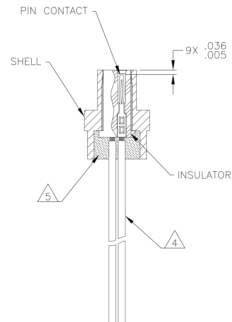
SECTION A-A
