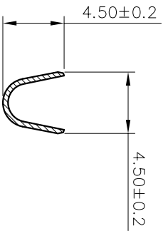
SECTION B-B 1:1
