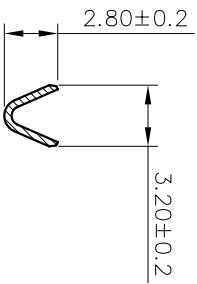
SECTION A-A 1:1
