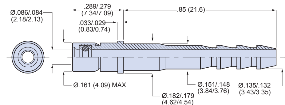
857-010 Socket Contact
