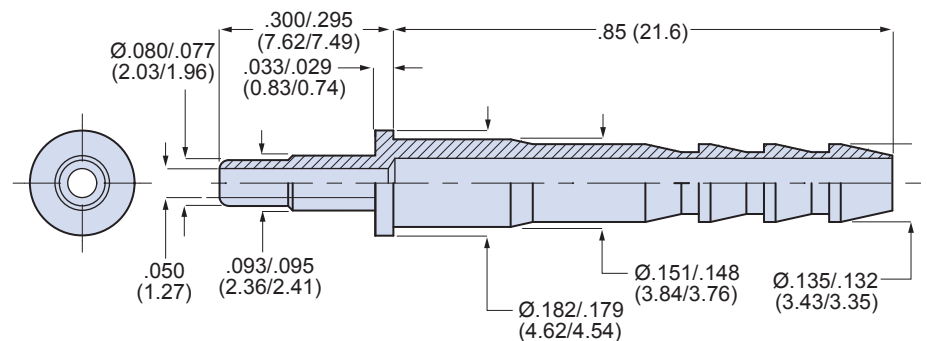
857-011 Pin Contact
