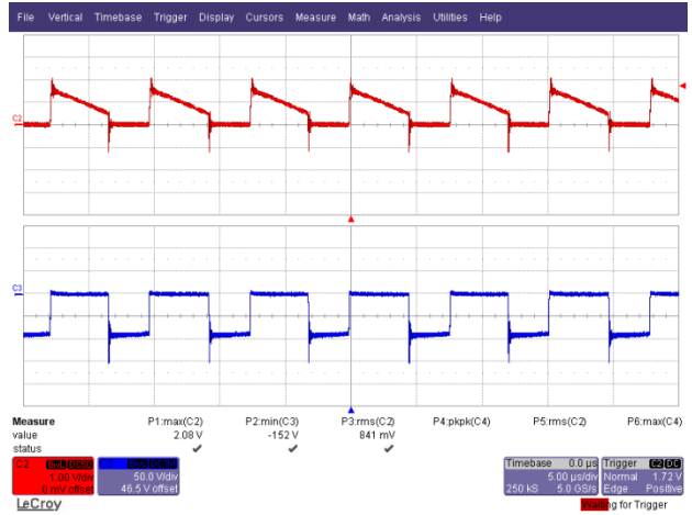
Figure 55 – 90 VAC, 60 Hz. Upper: I D5 , 0.2 A / div. Lower: V D5 , 50 V / div., 5 μs / div.
