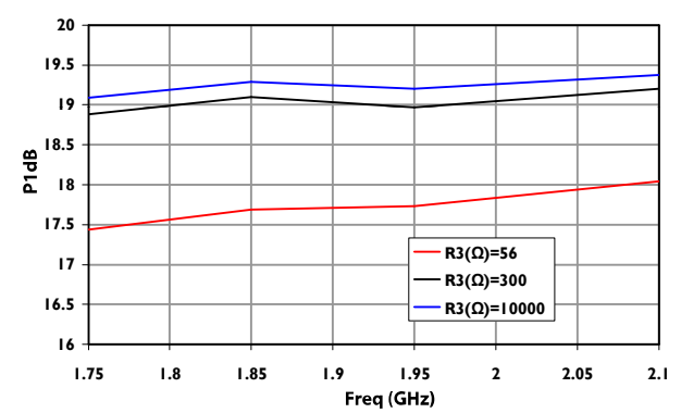
P1dB
