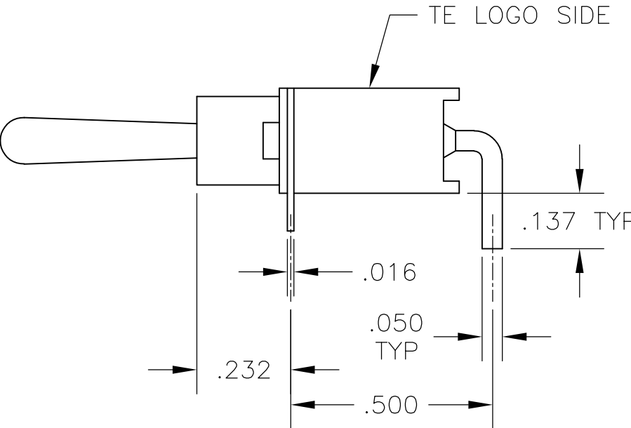
D1 BUSHING
