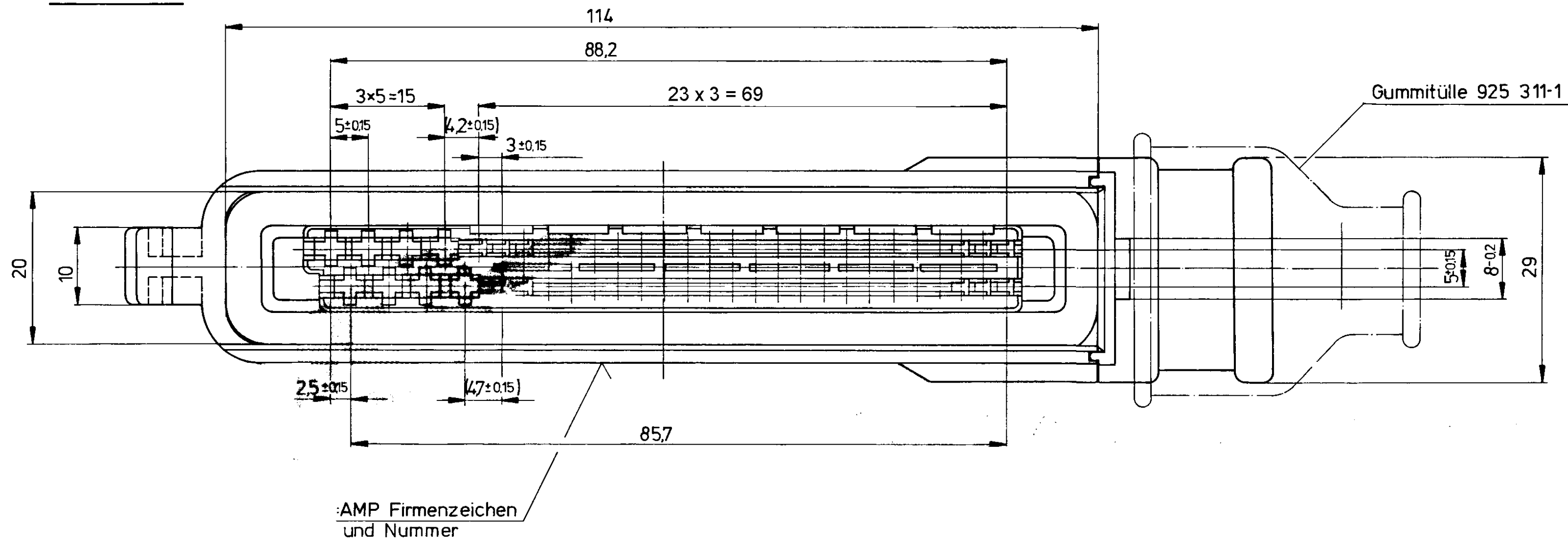
Ansicht X
