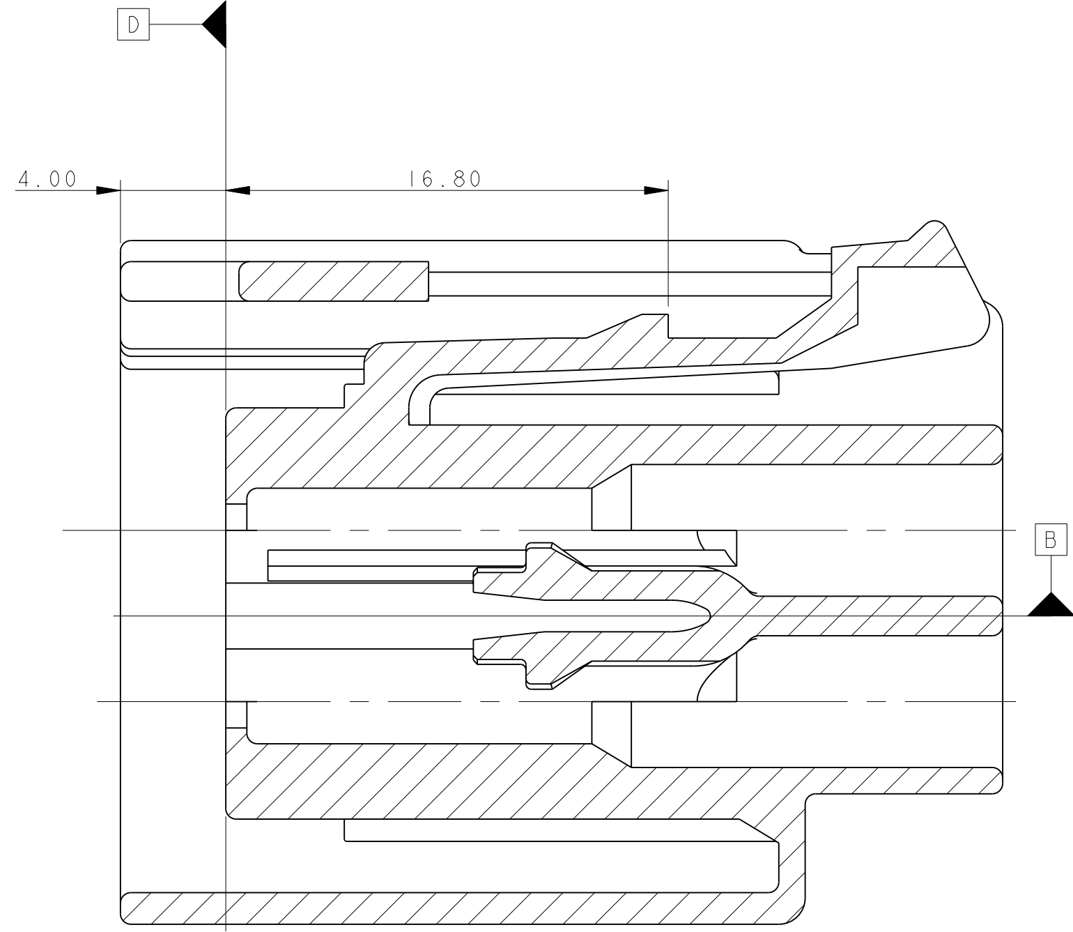
SECTION A-A
