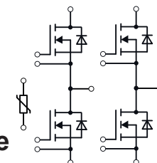
X112a E2-Pack PFP
