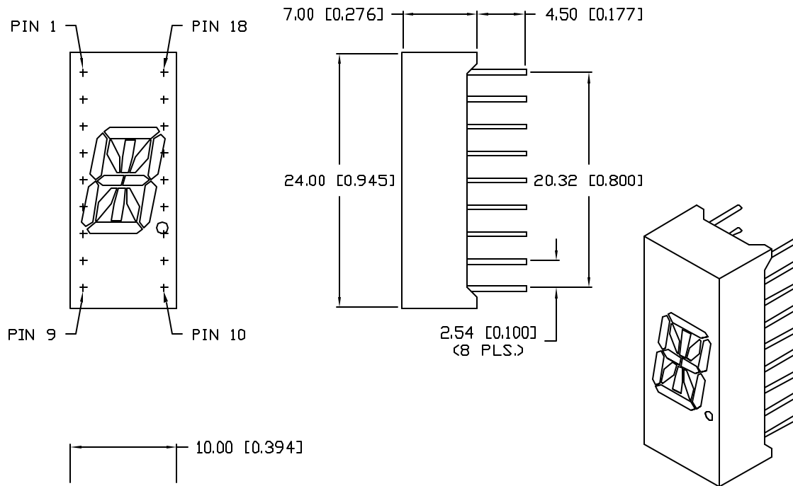
DIGIT DETAIL
