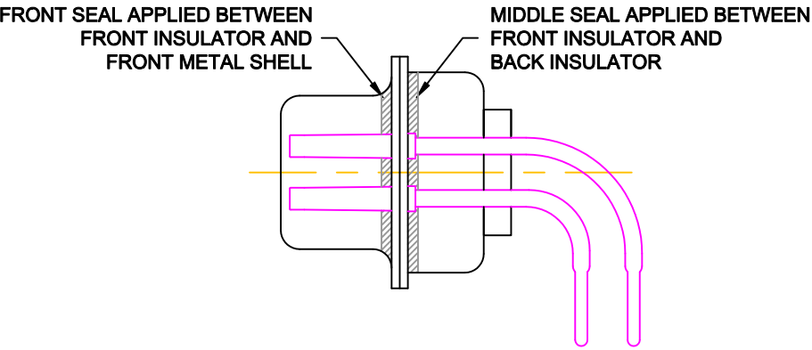
DETAIL A-A
