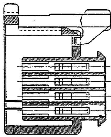
断面 A-A SECT.
