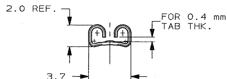
SEZIONE A-A (SECTION A-A)
