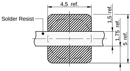
Scale - 5:1
