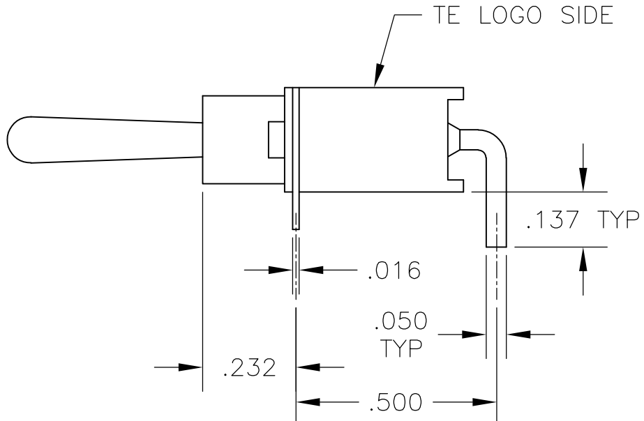
D1 BUSHING
