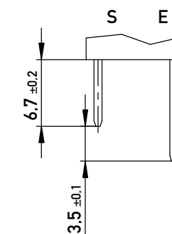
Stecklänge / mating length
