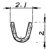
断面 B-B
