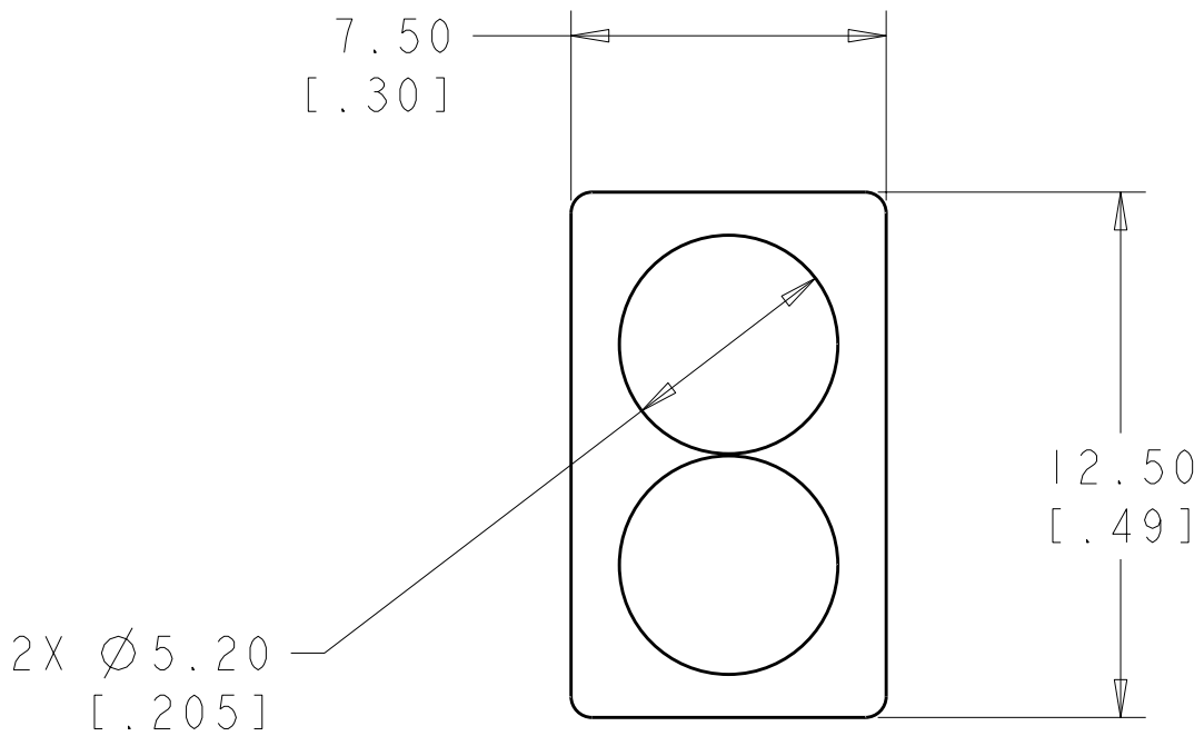
DETAIL ITEM 6 SCALE 5:1
