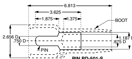
PIN PD-501-S
