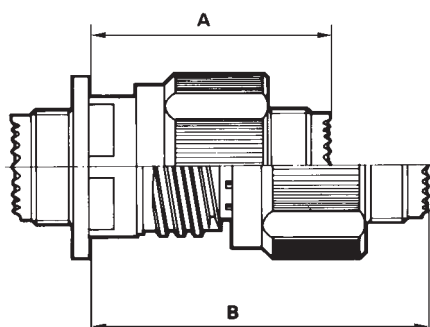
Type 0 avec fiche / Type 0 with plug
