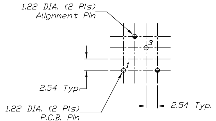
RECOMMEND P.C.B. LAYOUT
