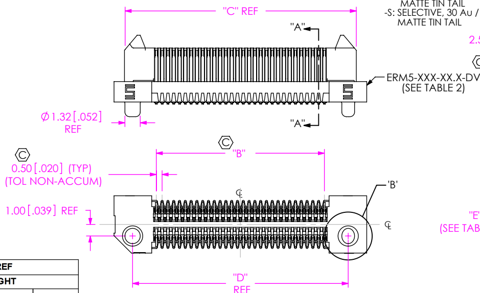
FIG 1 ERM5-030-02.0-X-DV-XX SHOWN
