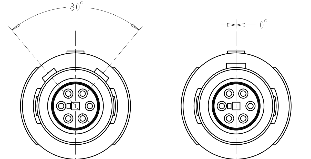
80° KEYING SCALE 4:1
