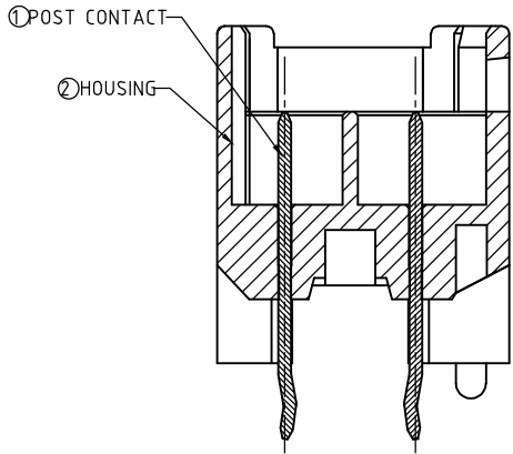
SECT A-A
