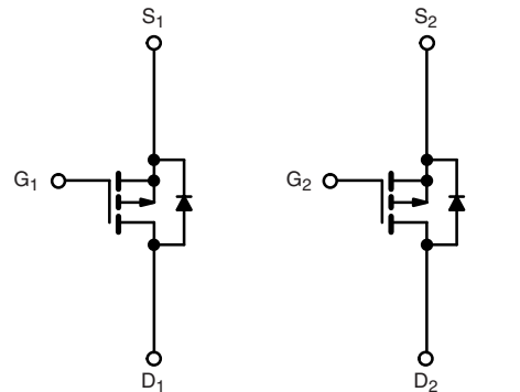
P-Channel MOSFET
