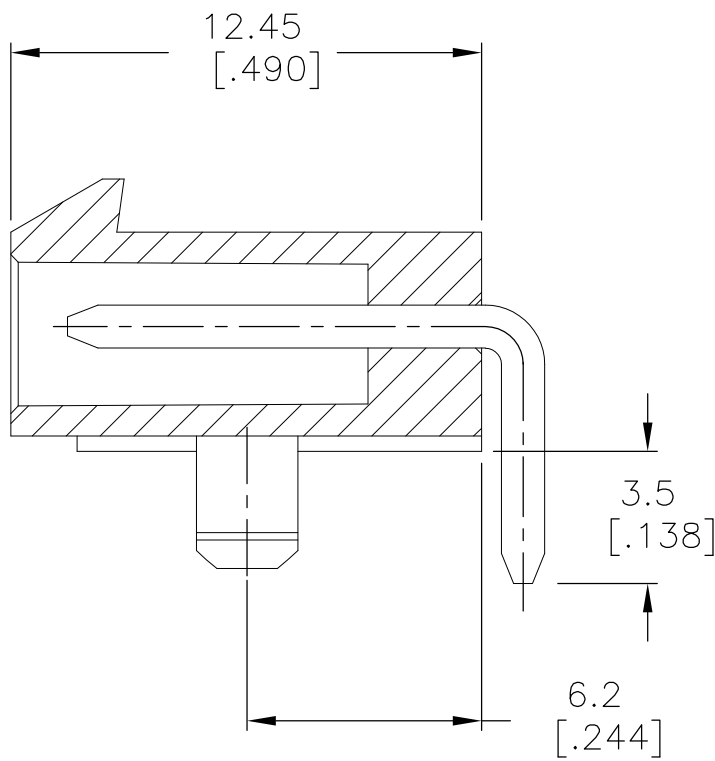
SECTION A-A
