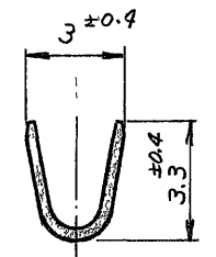
断面 A-A
