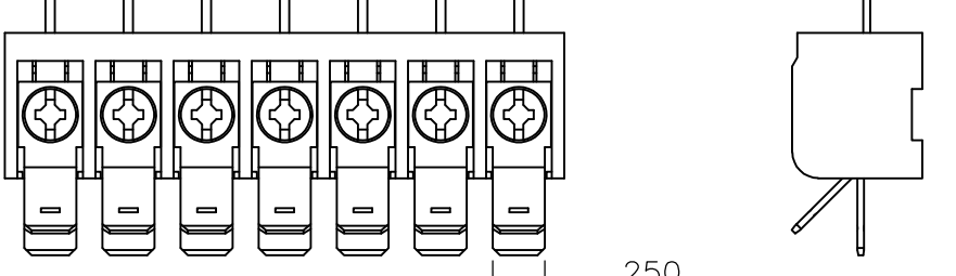
9-1437651-3 .250 TYP
