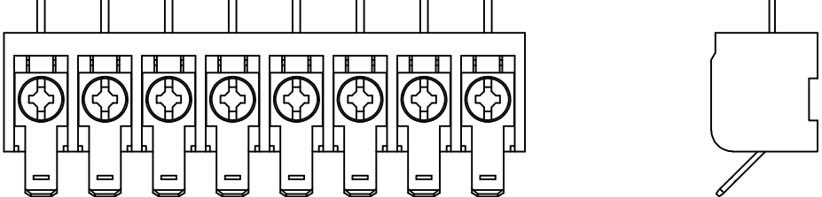
796905-1 .187 TYP
