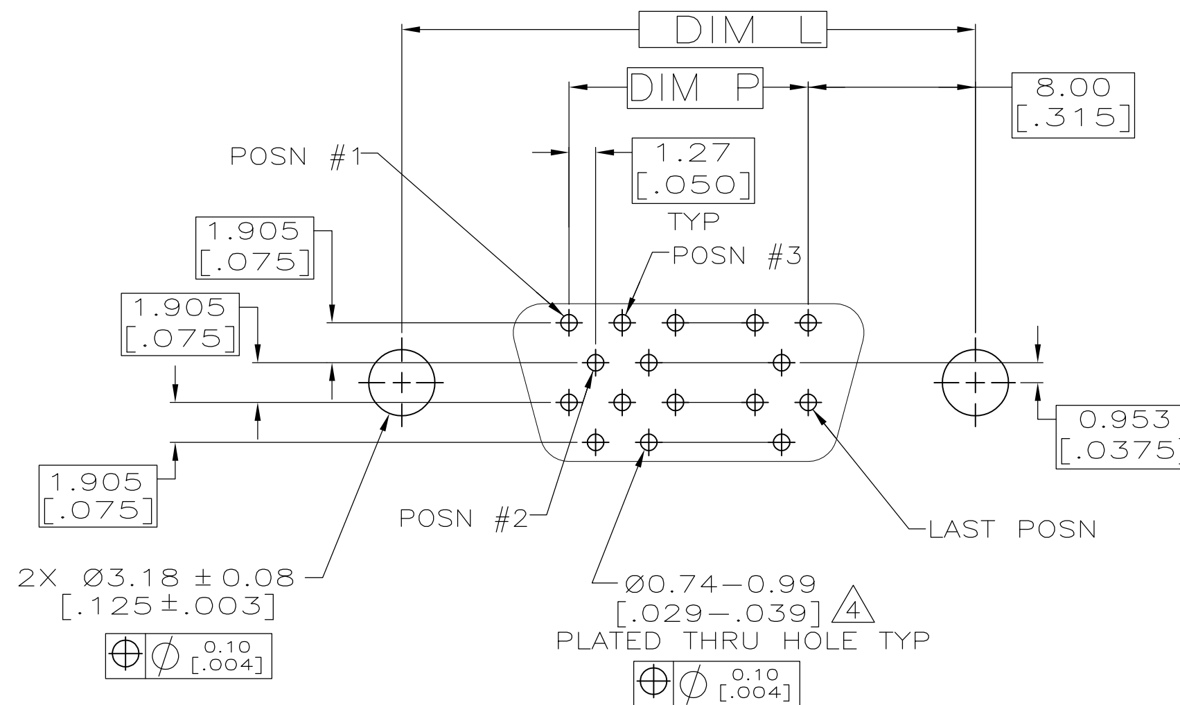
DETAIL Y
