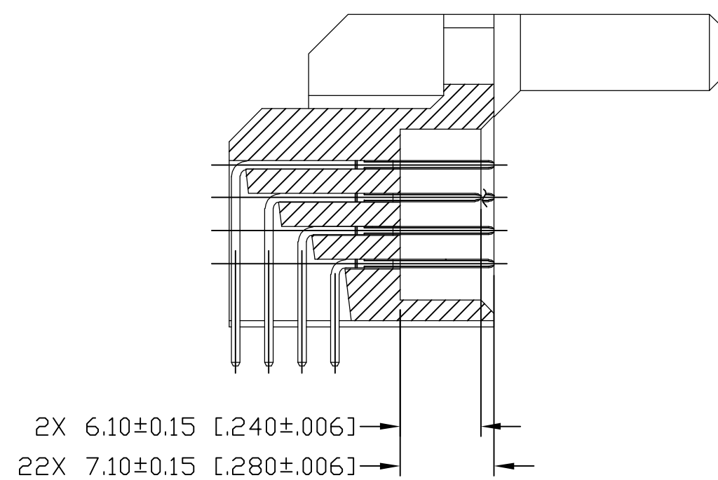
SECTION A-A SCALE: 2:1
