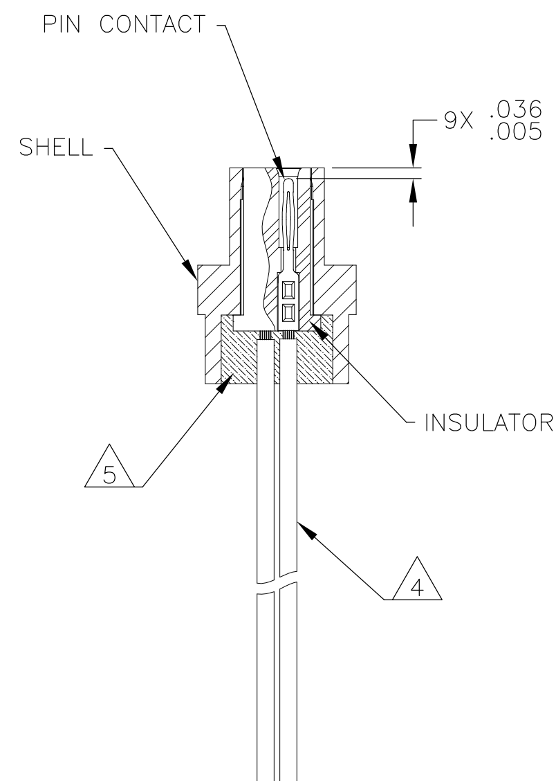
SECTION A-A
