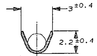
断面 C-C SECT. C-C
